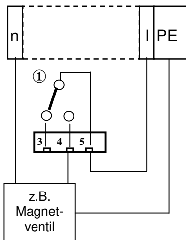
Anschlußbeispiel Grenzwertkontakt GW 1 schaltet Netzspannung
