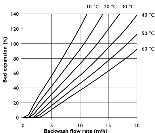
Fig. 1 : Bed Expansion
