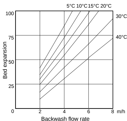
Fig. 1 : Bed Expansion
