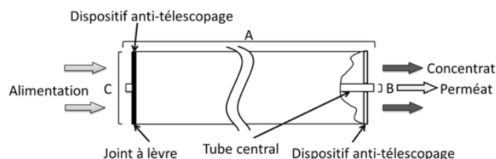
Figure 1a : Schéma d'encombrement de l'élément, côté mâle
