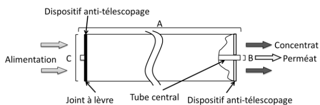
Figure 2 : Schéma des dimensions des éléments - mâles
