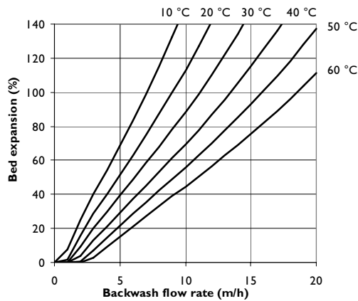
Fig. 1 : Bed Expansion
