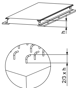
Fig. 29 Barre in acciaio come rinforzo nelle fondazioni
