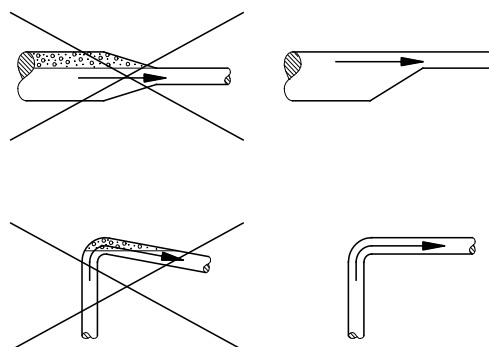
Fig. 31 Tubazioni
