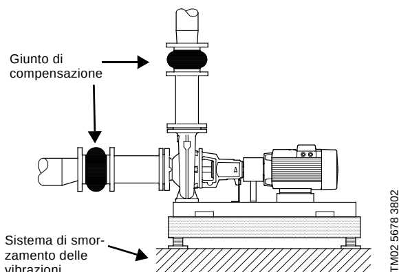
Fig. 33 Pompa NK con giunti ad espansione e smorzatori di vibrazioni
