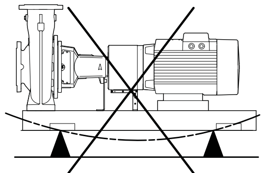
Fig. 27 Fondazione errata
