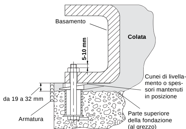
Fig. 30 Vista in sezione della fondazione con bullone, colata di malta e basamento
