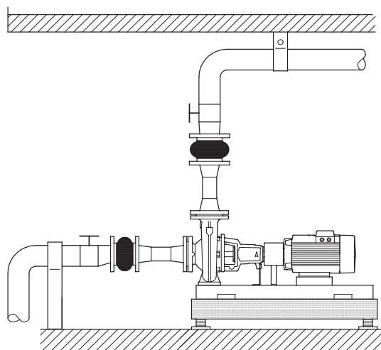
Fig. 32 Montaggio delle tubazioni
