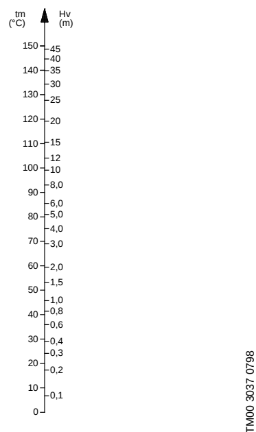
Fig. 24 Relazione tra temperatura del liquido e pressione del vapore
