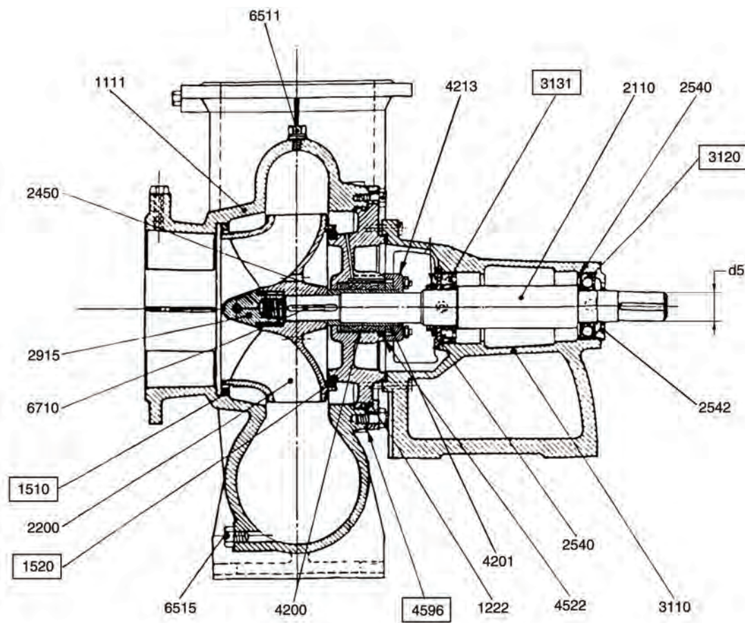
Fig. 7 Plano seccionado NK 200-400, 250-330, 300-360 "sobredimensionadas"
