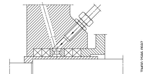
Fig. 18 Prensaestopas no refrigerado, tipo SNF(x), con líquido aislante externo para bombear líquidos contaminados y malolientes.
