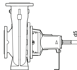
Fig. 26 Diámetro del eje libre d5
