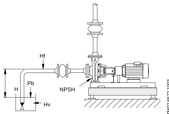
Fig. 28 Esquema de un sistema abierto con una bomba NK
