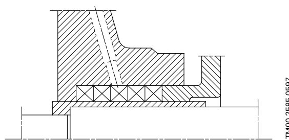
Fig. 17 Prensaestopas no refrigerado, tipo SNO(x), sin líquido aislante interno para bombear líquidos limpios en la aspiración o con presiones de entrada por encima de 4 bar.
