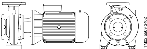
Fig. 8 Bomba NB, diseño A
