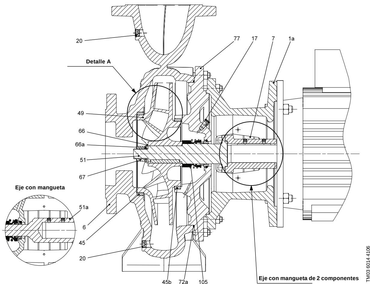
Fig. 3 Plano seccionado NB
