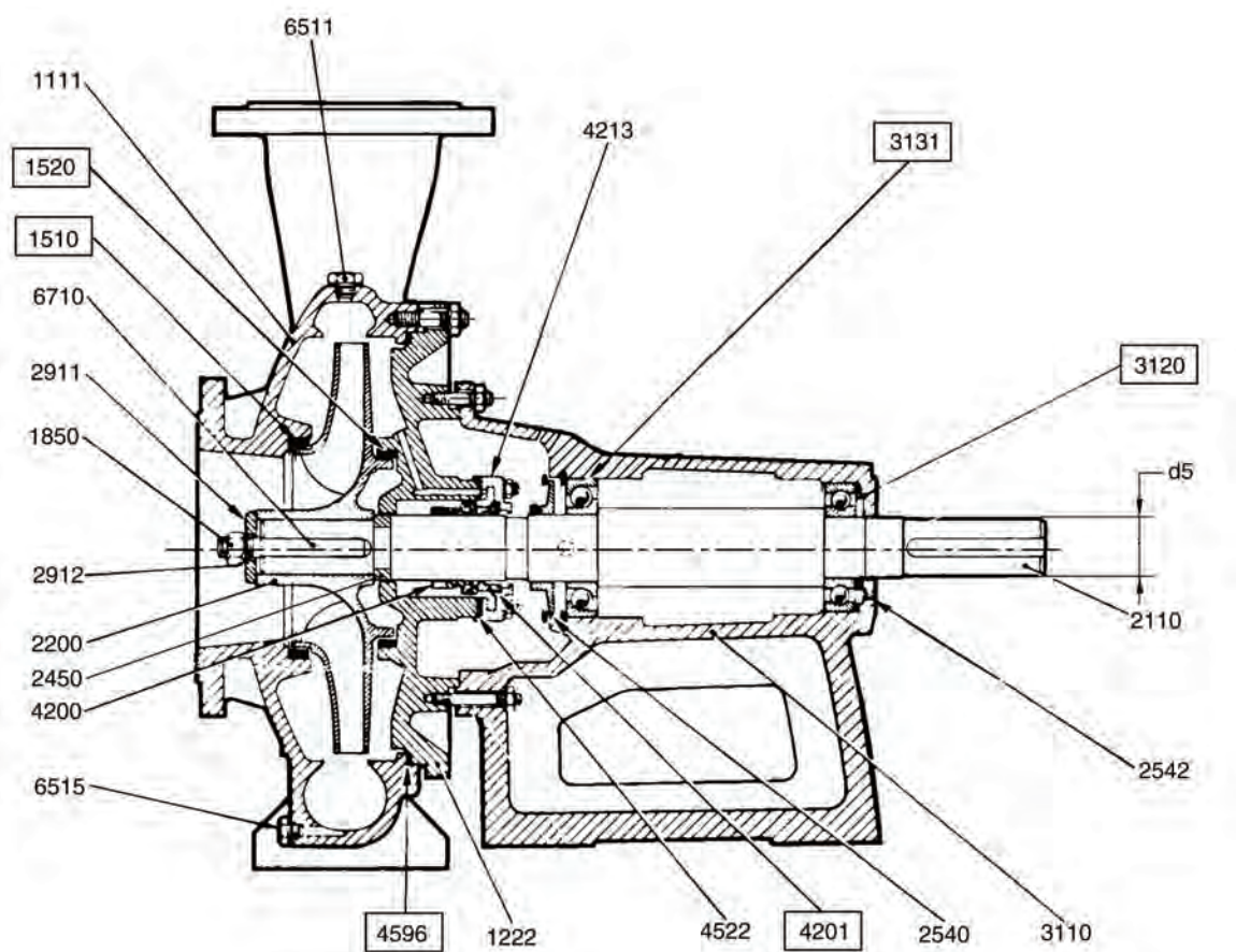
Fig. 6 Plano seccionado, NK 200-500, 250-400, 250-500 "sobredimensionadas"
